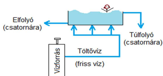
1. ábra: Töltő-ürítő technológiával üzemelő medence vázlata 2
